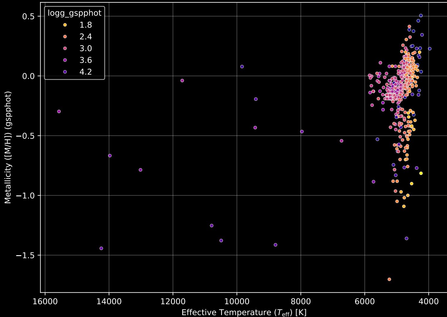
APOGEE DR17 Field: [100-06] Stellar Population Parameters (n= 444)
